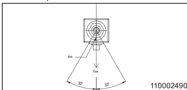
Schéma du capteur monté dans un tuyau
